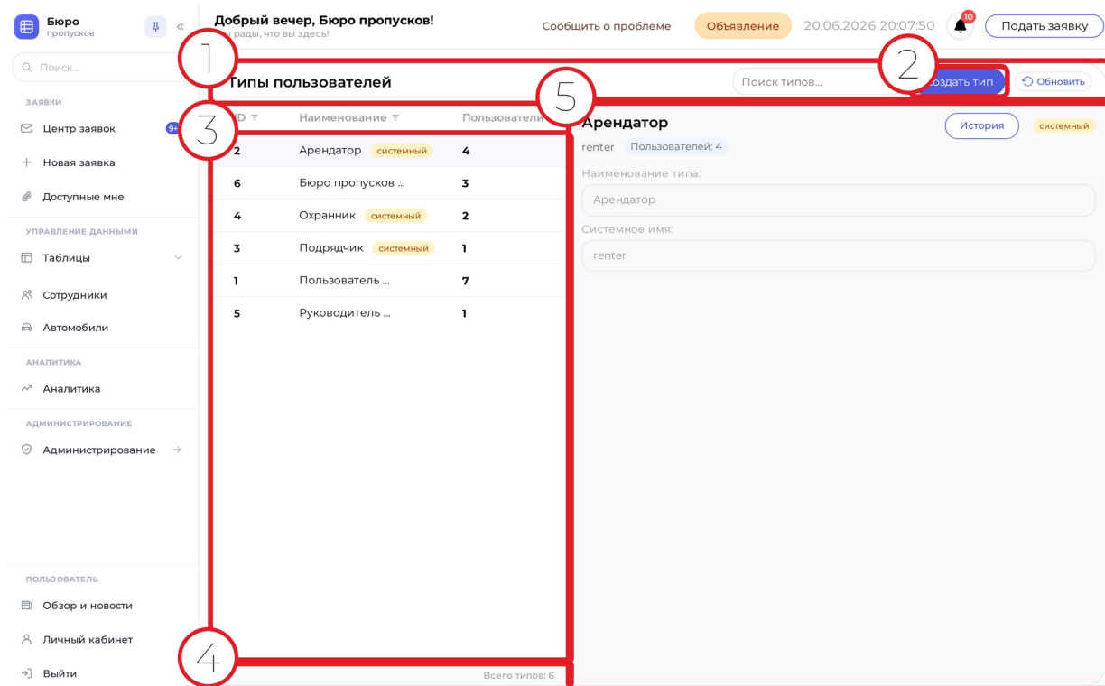
Рисунок 15 — Типы пользователей
